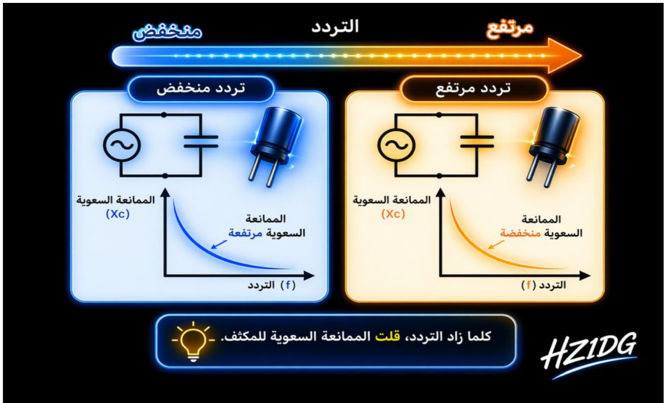
شكل (٥-٦): تغير الممانعة السعوية للمكثف مع التردد.
