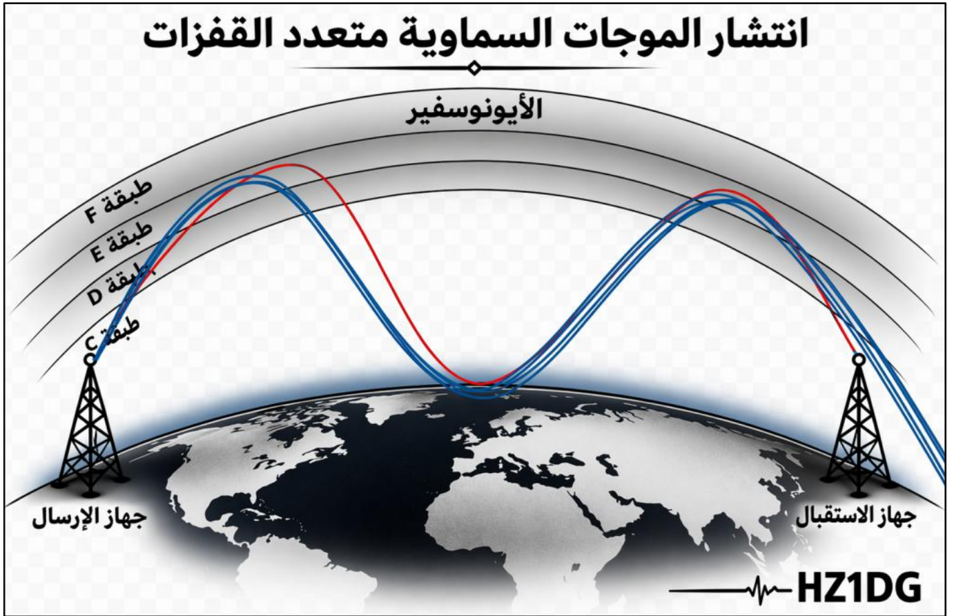
شكل (٤-٥) : القفزات المتعددة للموجة
