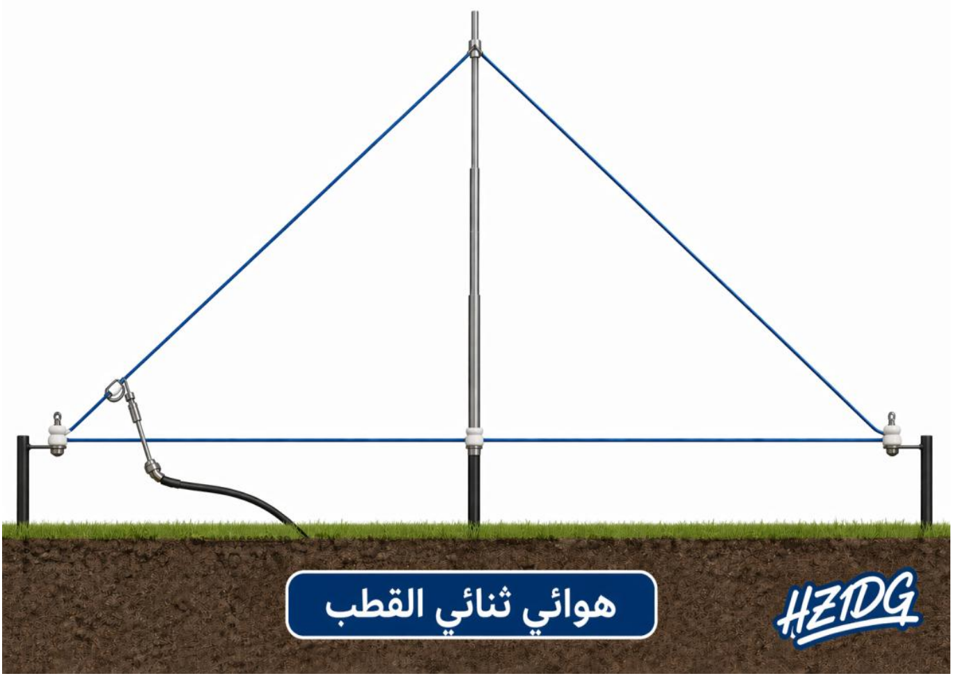
شكل (٤-٨): هوائي Dipole
