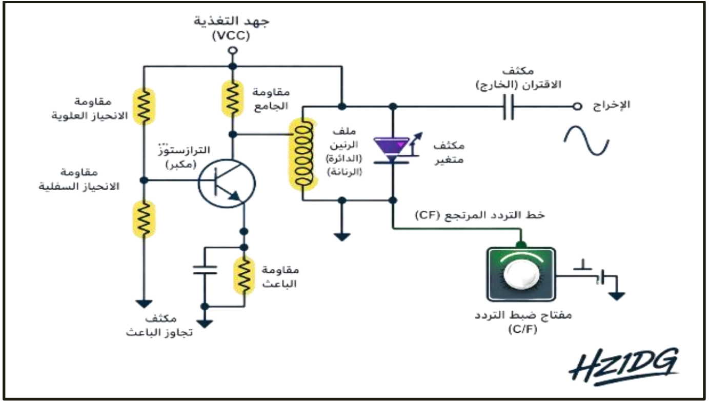
شكل (٩-٦): مذبذب متحكم بالجهد (VCO)
