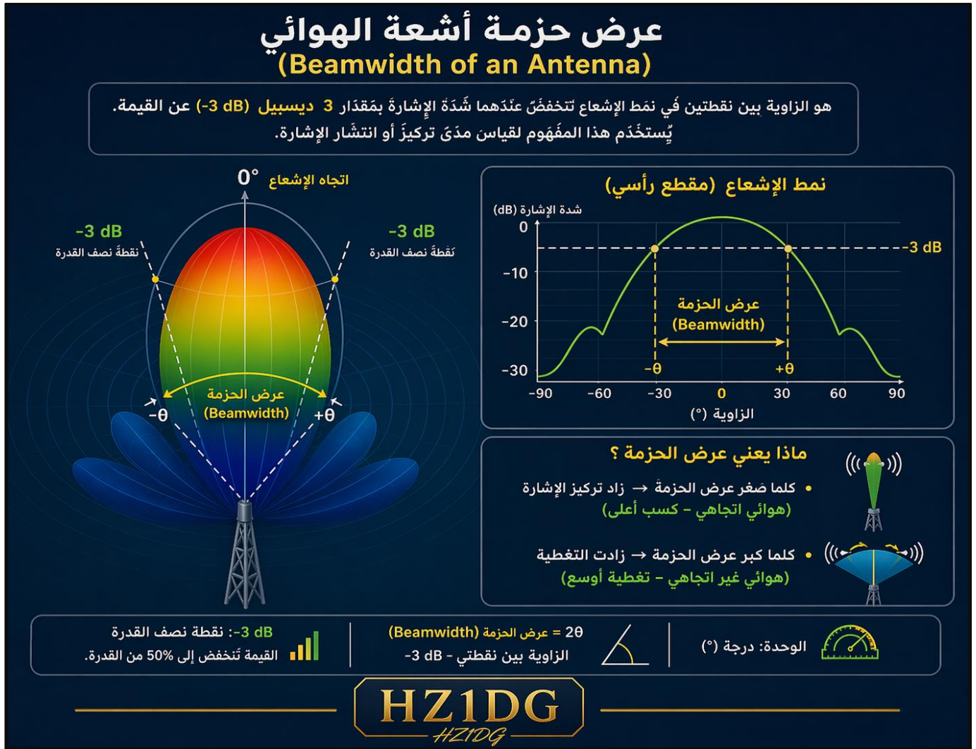
شكل (٨-١٠): عرض حزمة أشعة الهوائي
