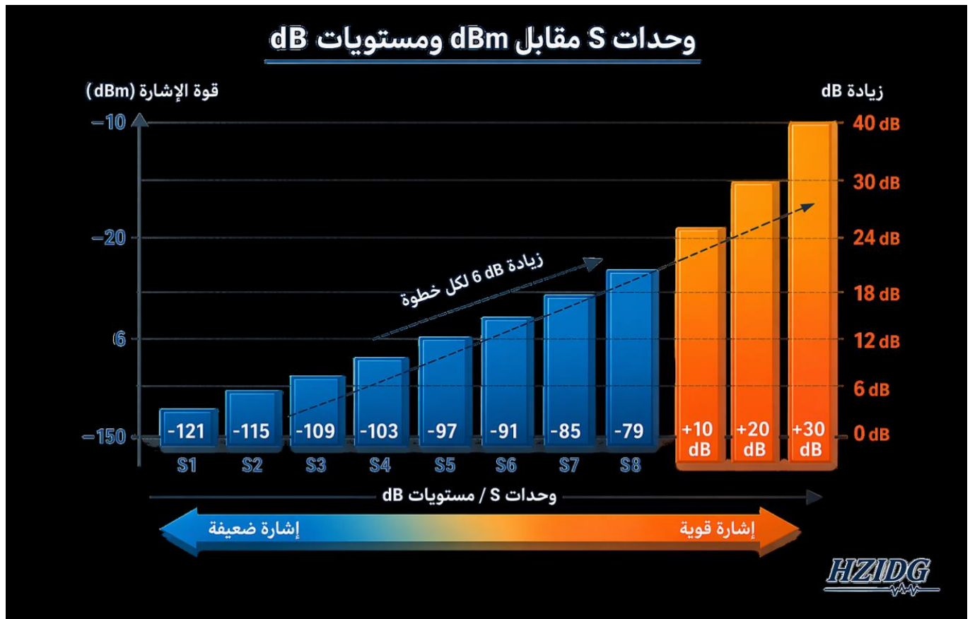
شكل (١٠-٧): رسم بياني لمقياس الإشارة بعد S9 (S-Meter + dB)
