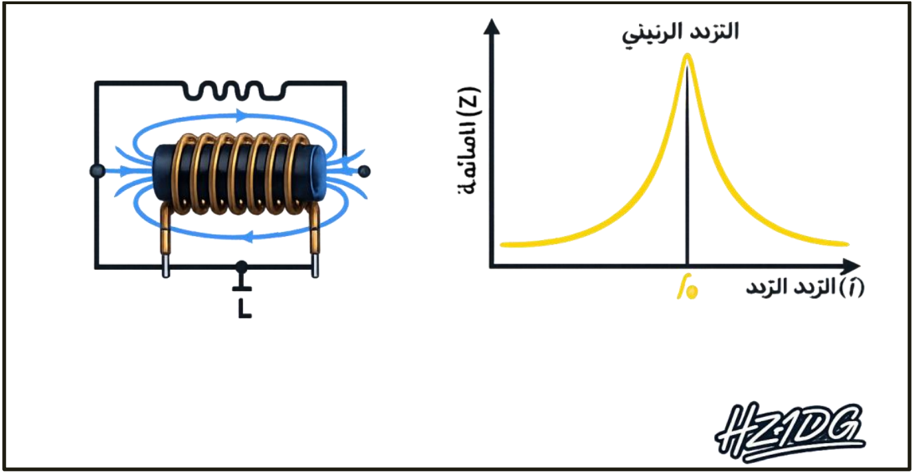
شكل (٦-٨): منحني الرنين وعلاقته بالتردد
