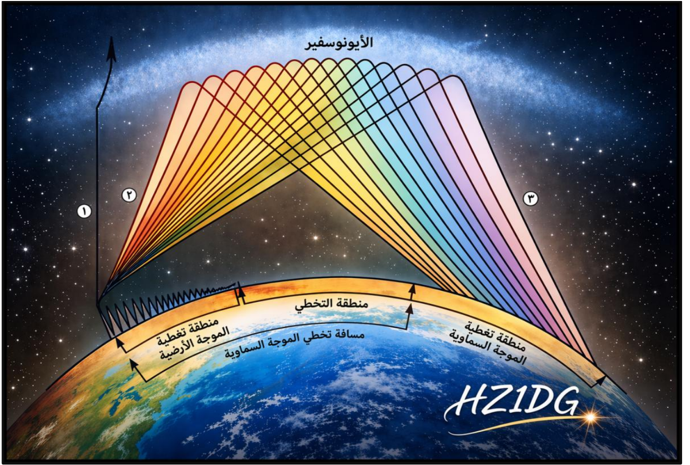
شكل (٣-٥): توضيح المسافة الصامتة (Skip Distance)
