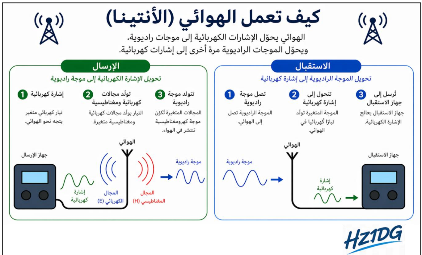
شكل (١-٨): مبدأ عمل الهوائي
