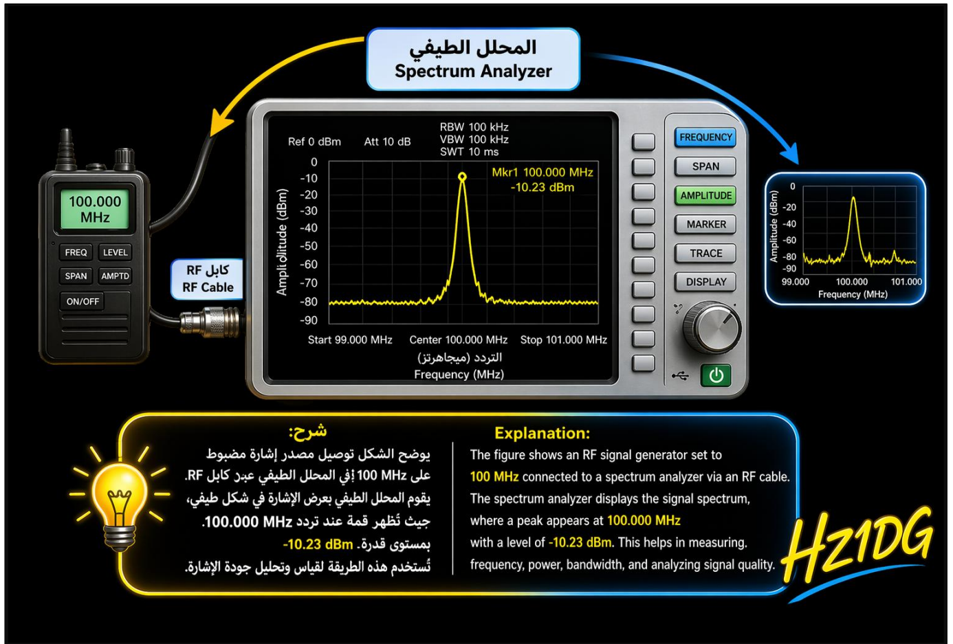
شكل (١٤-٦): عرض الإشارة باستخدام المحلل الطيفي (Spectrum Analyzer)
