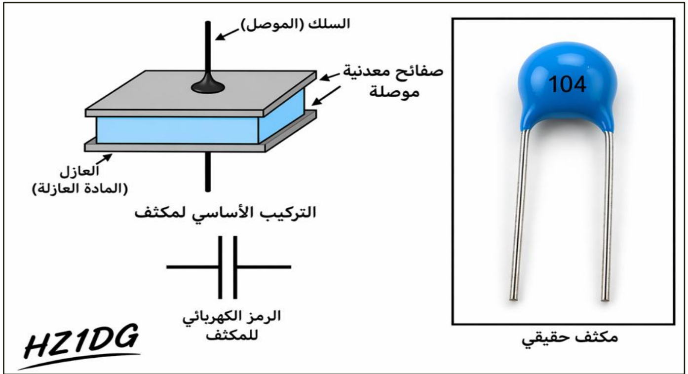
شكل (٤-٦): البنية الأساسية للمكثف وتمثيله الرمزي.
