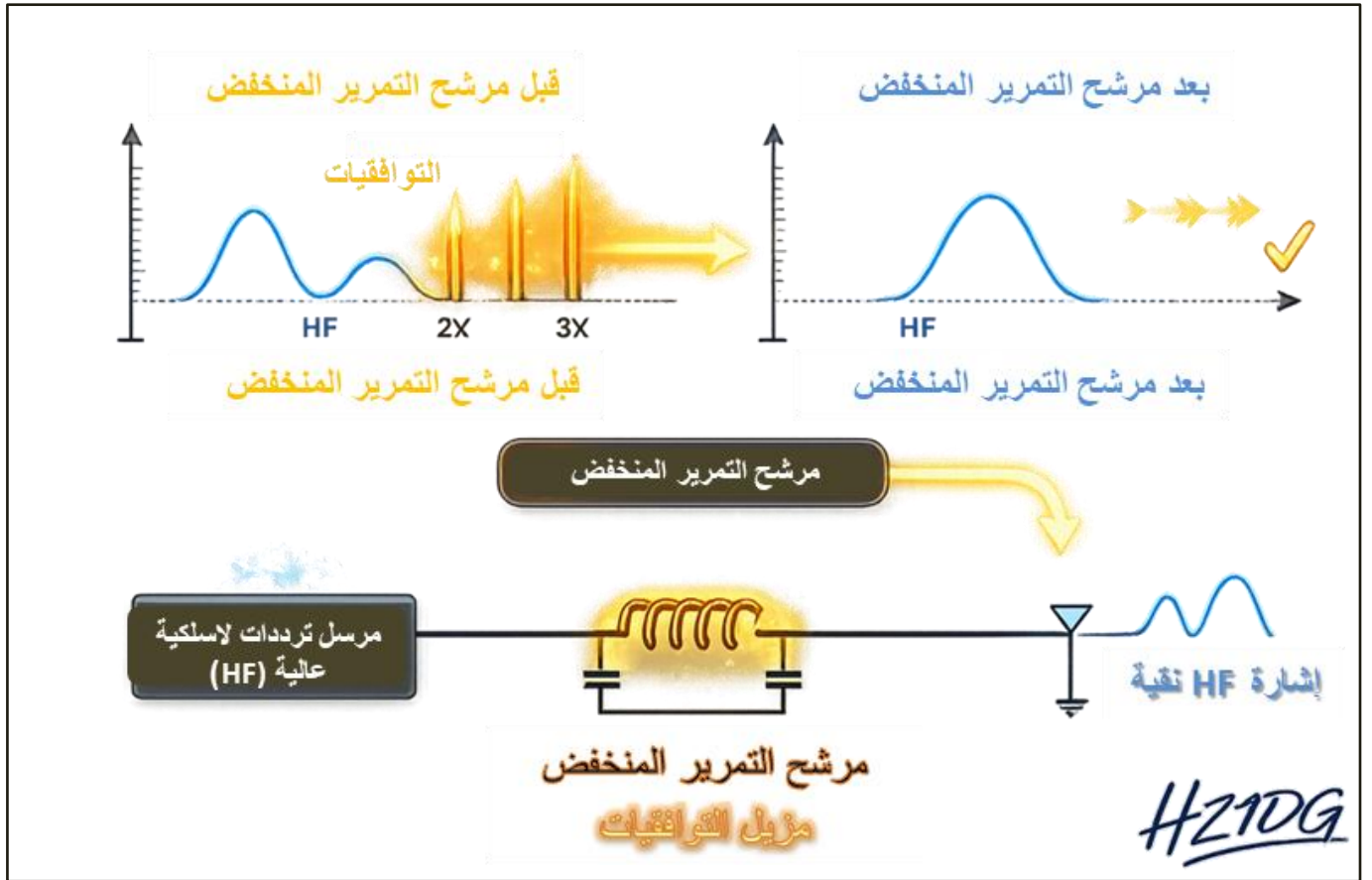
شكل (١٠-٦): تأثير المرشح منخفض التمرير (Low-Pass Filter) على الإشارة وإزالة التوافقيات
