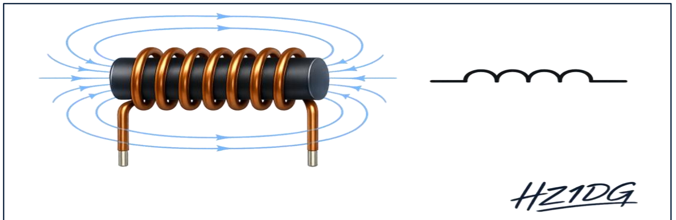
شكل (٦-٦): الملف (Inductor) والمجال المغناطيسي حوله ورمزه.
